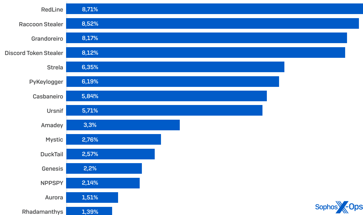
Figura 6: I rilevamenti di malware di tipo info stealer nel 2023, tratti dai dati di telemetria dei clienti Sophos raccolti dai SophosLabs
