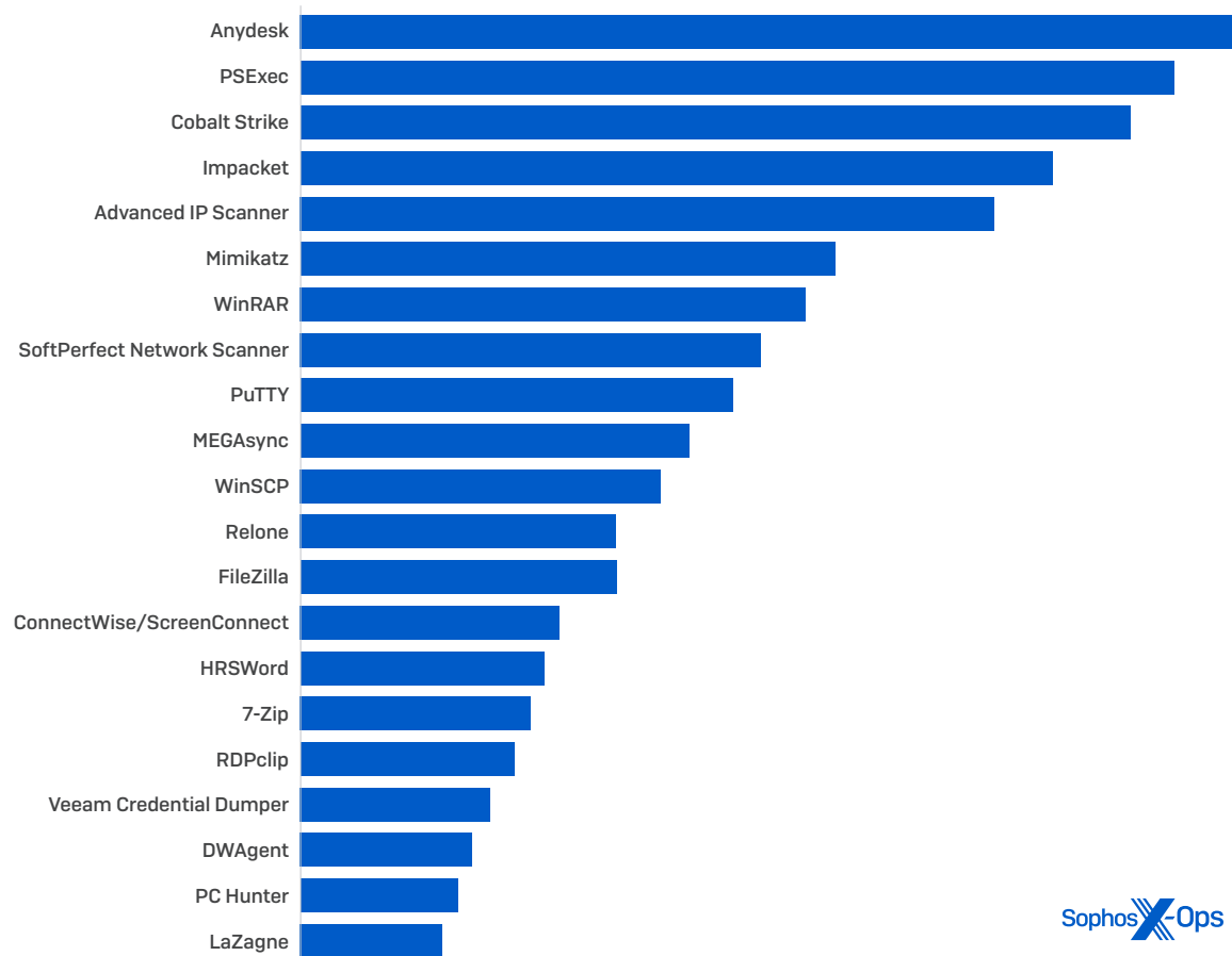
Figura 12: Gli strumenti “a duplice applicazione” più frequentemente osservati negli incidenti di sicurezza, in base al numero di casi in cui ciascuno di essi è stato osservato nei dati di Sophos MDR
