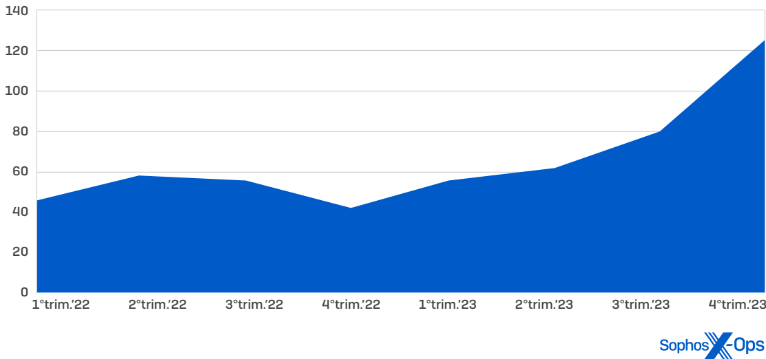
Figura 10: Gli ultimi due anni di dati di telemetria dei clienti raccolti da Sophos indicano un incremento generale nella percentuale di tentativi di attacchi ransomware che includono il remote ransomware: un problema attuale che si è ripresentato con maggiore insistenza, specialmente nella seconda metà del 2023
