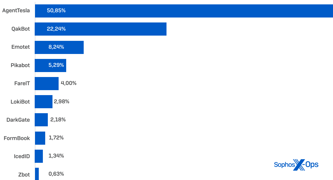
Figura 11: Una ripartizione dei framework più comunemente utilizzati dagli autori degli attacchi per distribuire il malware, in base al numero di rilevamenti su endpoint effettuati nelle reti dei clienti protetti con Sophos; le statistiche di QakBot rappresentano i rilevamenti prima dell'intervento internazionale delle forze dell'ordine contro l'infrastruttura di questa minaccia, avvenuto ad agosto 2023
