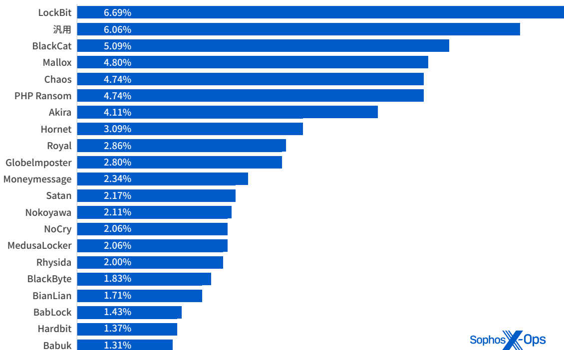
図 8：2023 年に Sophos Endpoint Protection ソフトウェアによって検出され、Labs データセットに存在するランサムウェア展開の試行件数の上位を、検出されたランサムウェア全体に占める割合で示したもの。「Generic」とは、別の定義では検出されなかったが包括的シグネチャで検出されたさまざまな種類のランサムウェアを示す
